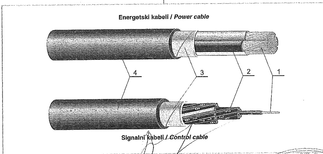
Slika 2. Konstrukcija kabela tipa NYY i NAYY
