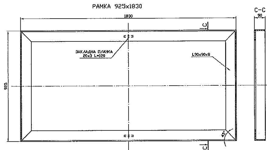
Фиг. 1 – Размери на метални рамки за капаци за кабелни шахти
