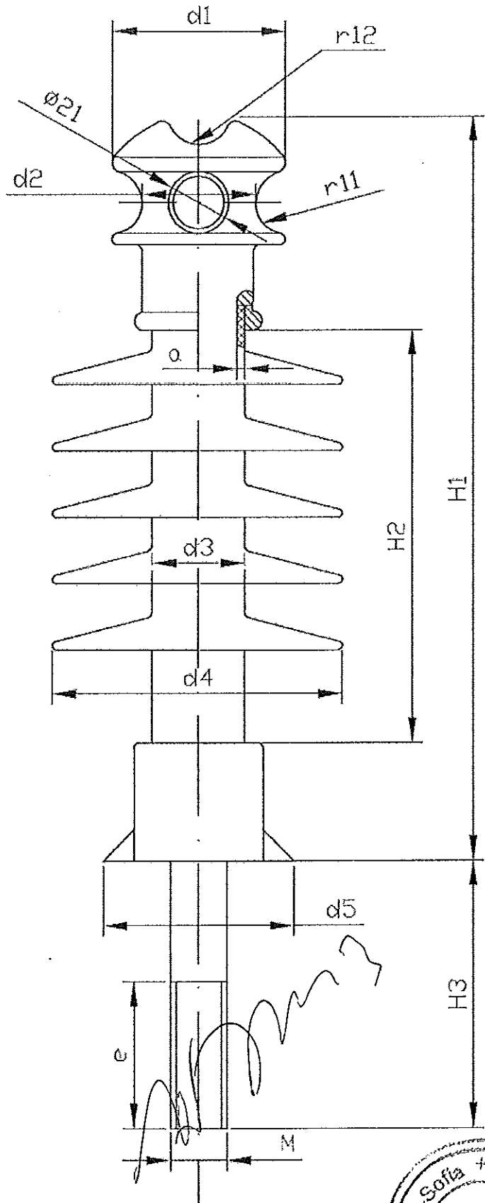
Фигура 1 - Носец композитен изолатор 20 kV
