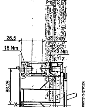
Front for copper/aluminium cables - FC CuAl 300 mm 2
