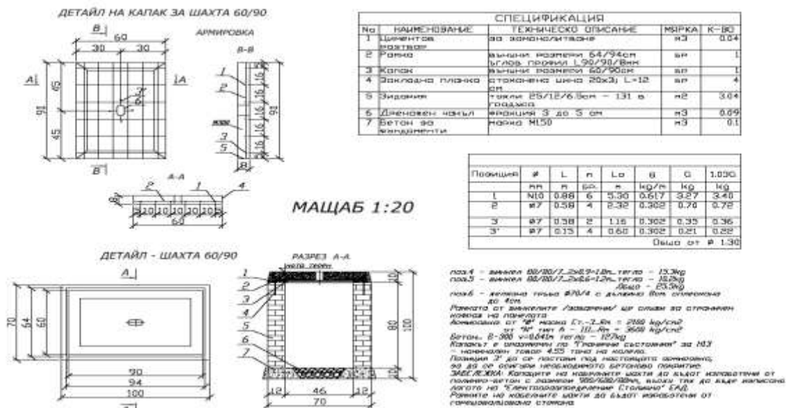
Фиг. 1. Кабелна шахта – единичн
