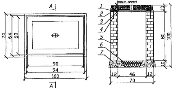
ДЕТАЙЛ - ШАХТА 60/90
