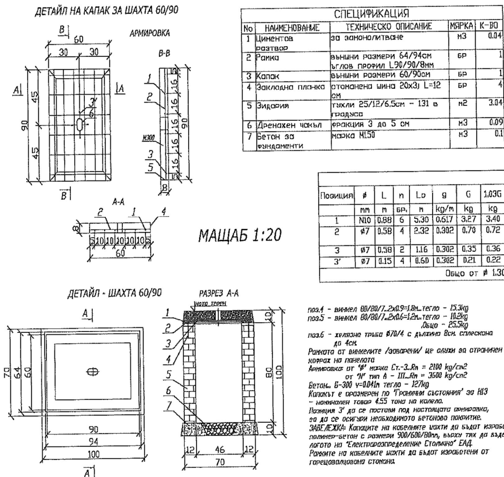
Фиг.6.3. Кабелна шахта – единична
