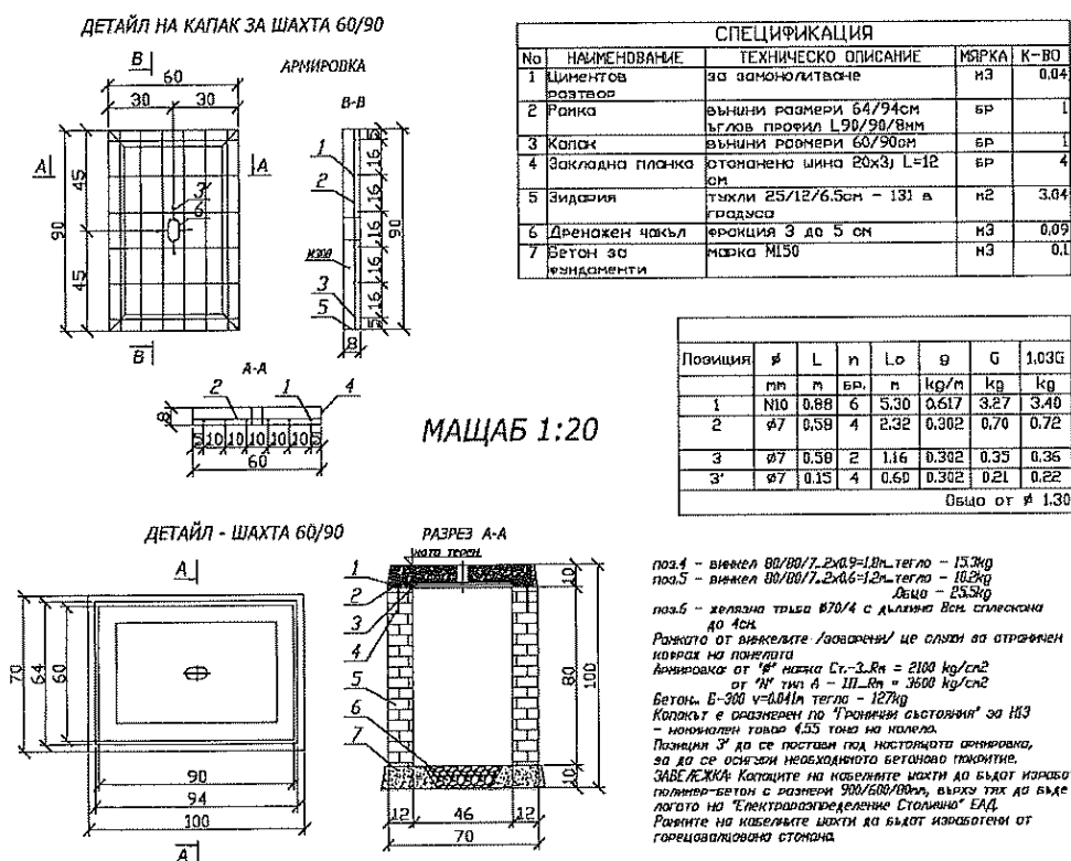
Фигура - Кабелна шахта – единична
