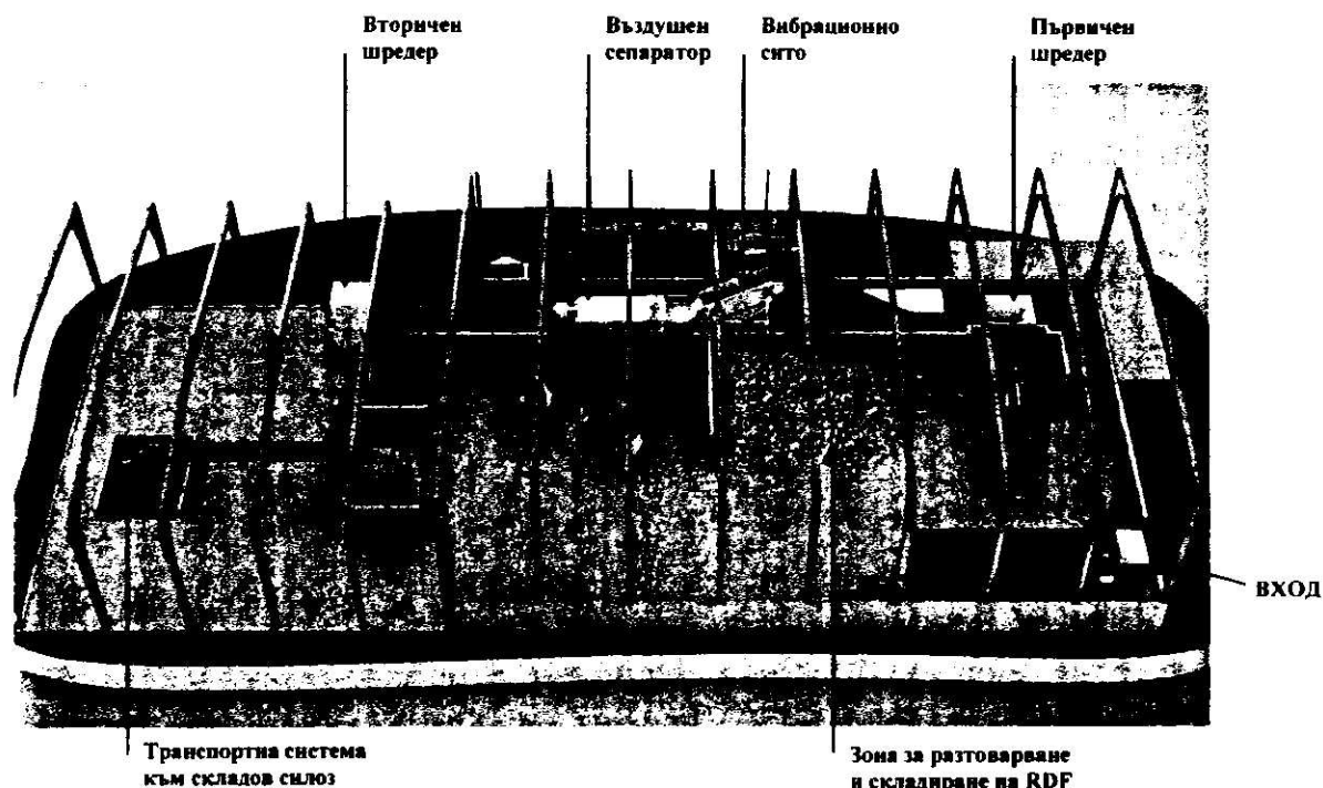
Фиг. 1: Ген-план на инсталацията със схема за разтоварване и складиране
