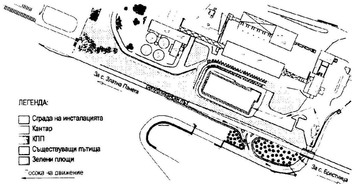
Фиг. 2: Ген-план на завода със схема за транспорт
