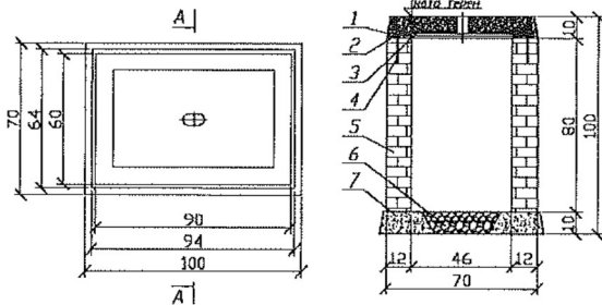
ДЕТАЙЛ - ШАХТА 60/90
