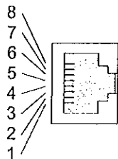
Рис. 18 – RS-232, RS-485, GPS
