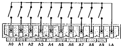
Рис. 39 – Активни DI
