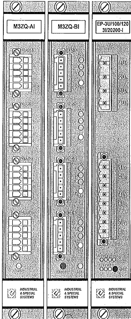
Fig. 61 - RTU7M-M3ZQ-AI, RTU7M-M3ZQ-BI, RTU7M-EP
