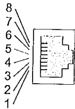
Рис. 65 - Конектор RJ45 интерфейс RS-485
