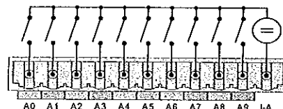
Рис. 44 – Пасивни DI
