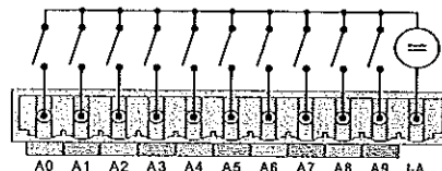
Рис. 40 – Пасивни DI
