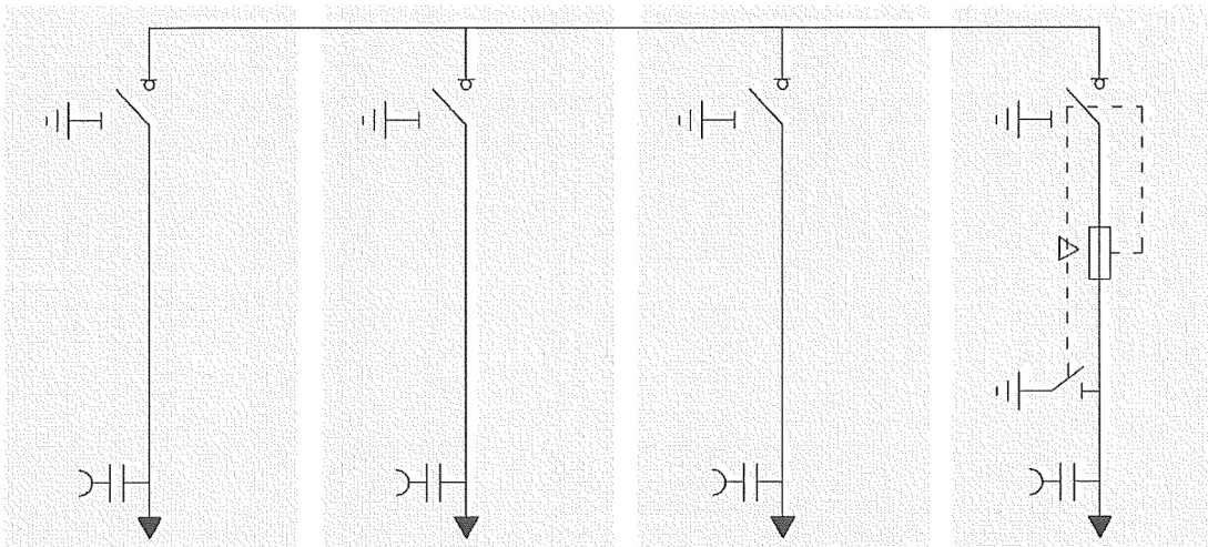
4.10 Комплектна разпределителна уредба в метални шкафове 12 kV, 630 A, 16 kA с SF 6 товари прекъсвачи – три кабелни присъединения и едно трансформаторно присъединение
