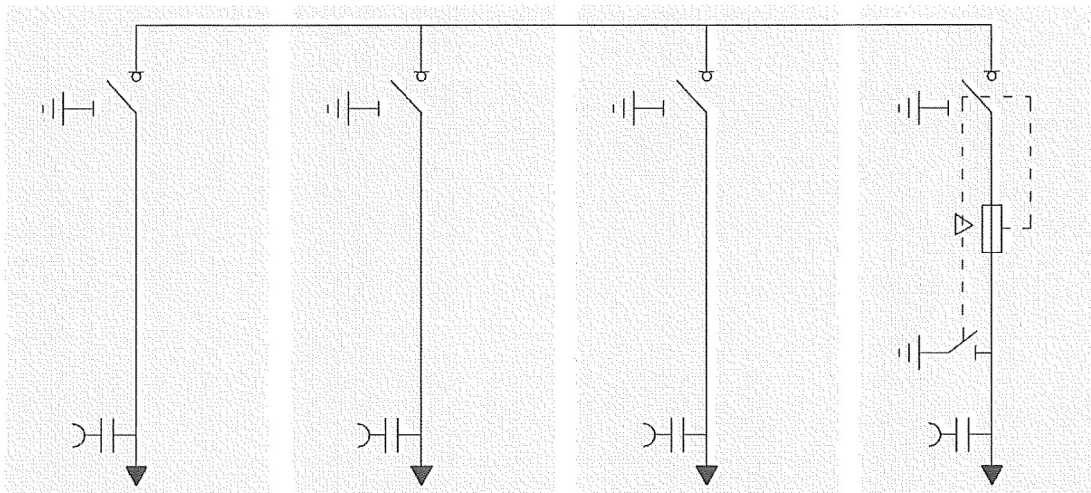
4.11 Комплектна разпределителна уредба в метални шкафове 24/25 kV, 630 A, 16 kA с SF 6 товарови прекъсвачи – две кабелни присъединения и две трансформаторни присъединения
