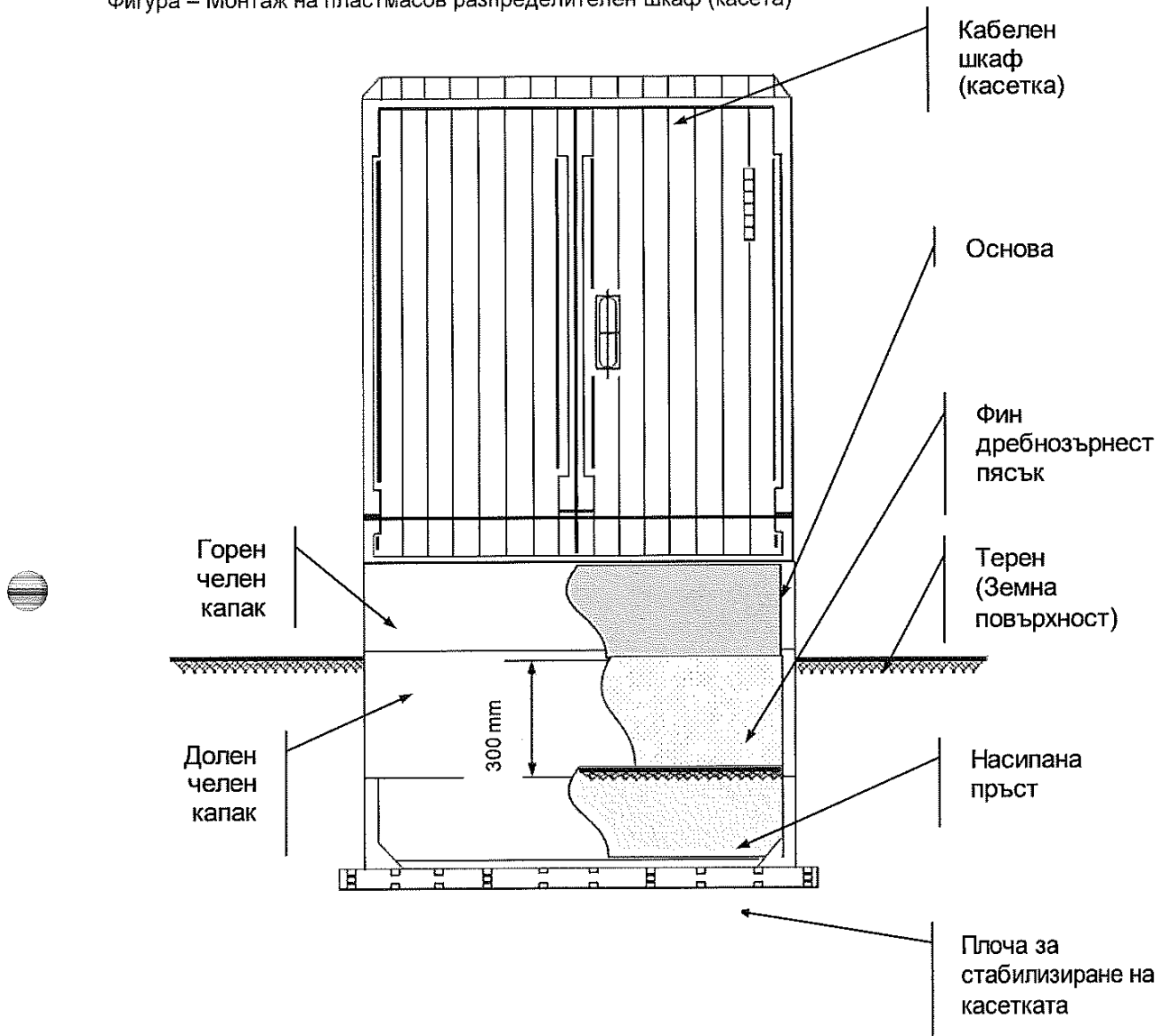
Фигура – Монтаж на пластмасов разпределителен шкаф (касета)
