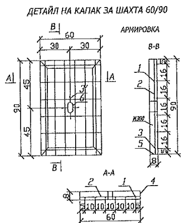
Фиг.6.3. Кабелна шахта – единична
